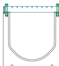
Sistemi di fissaggio tra canalette e griglie MAGNUM CITY / Lock system between MAGNUM CITY channels and gratings
