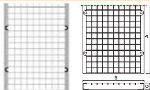
Griglia a maglia 30x30 acciaio zinc./inox Mesh 30x30 grating galvanized/s. steel
