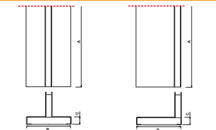
Griglia a fessura acciaio zincato Galvanized Shaped Grating Disponibile a richiesta / Available on request
