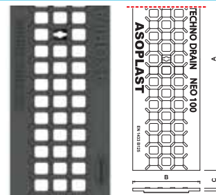
Griglia a maglia ghisa sferoidale Ductile iron mesh grating
