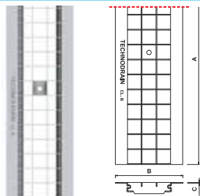
Griglia a maglia 30x30 acciaio zinc./inox Mesh 30x30 grating galvanized/s.steel
